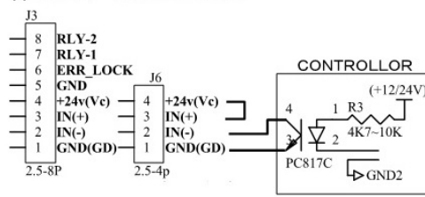
(7) 接地隔離 - NPN型配線參考圖
