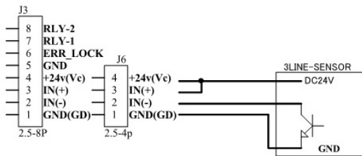
(3) Sensor - PNP型配線參考圖
