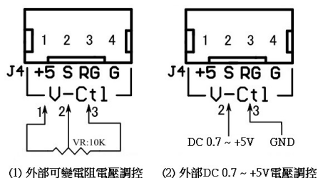
(1) 外部可變電阻電壓調控 (2) 外部DC 0.7 ~ +5V電壓調控
