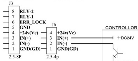
(7) 接地隔離 - NPN型配線參考圖
