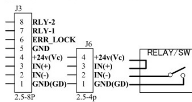
(6) 接地隔離 - 光耦合配線參考圖
