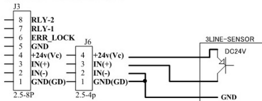
(3) Sensor - PNP型配線參考圖
