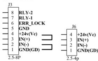
(2) Sensor - NPN型配線參考圖
