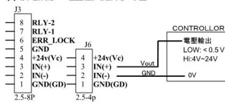
(8) 接地隔離 - 電壓輸出配線參考圖
