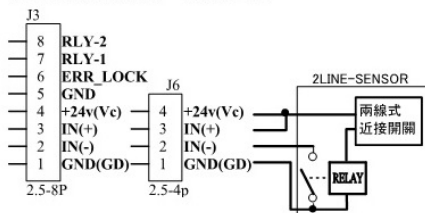
(4) 兩線式近接開關 - 配線參考圖
