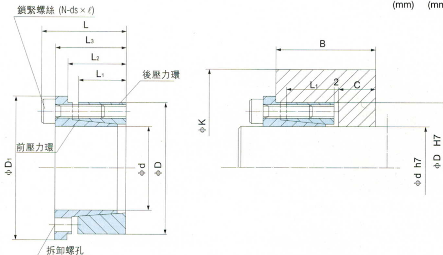
尺寸、性能 輪殼內徑表面受面壓 (P B ) 時的必要最小外徑 \phi K (B \geq 2 \times L_1, C \geq \frac{1}{2})
